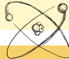
Méson
